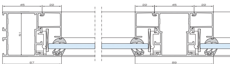
Przekrój poziomy przez witrynę ze stałym szkleniem
