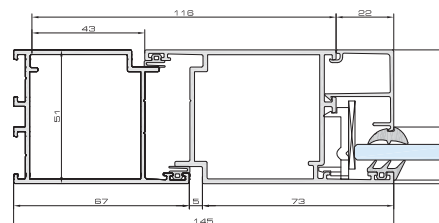
Przekrój poziomy przez ramę drzwi otwieranych do wewnątrz
