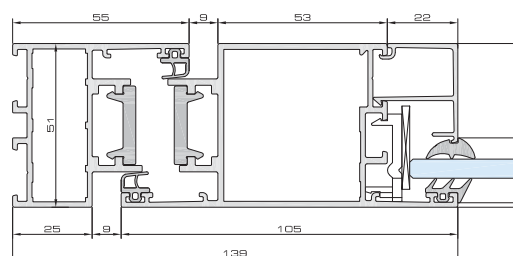
Przekrój poziomy przez ramę drzwi otwieranych na zewnątrz
