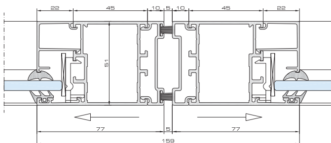
Przekrój poziomy przez słupek środkowy drzwi przesuwnych
